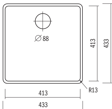
FSP-44 413 x 413 x 210mm R13
